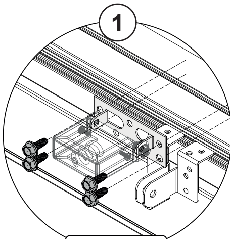
1 C9958/ C9959
